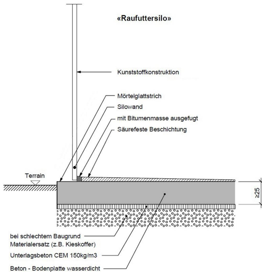
Kunststoffsilo (Beispiel)
